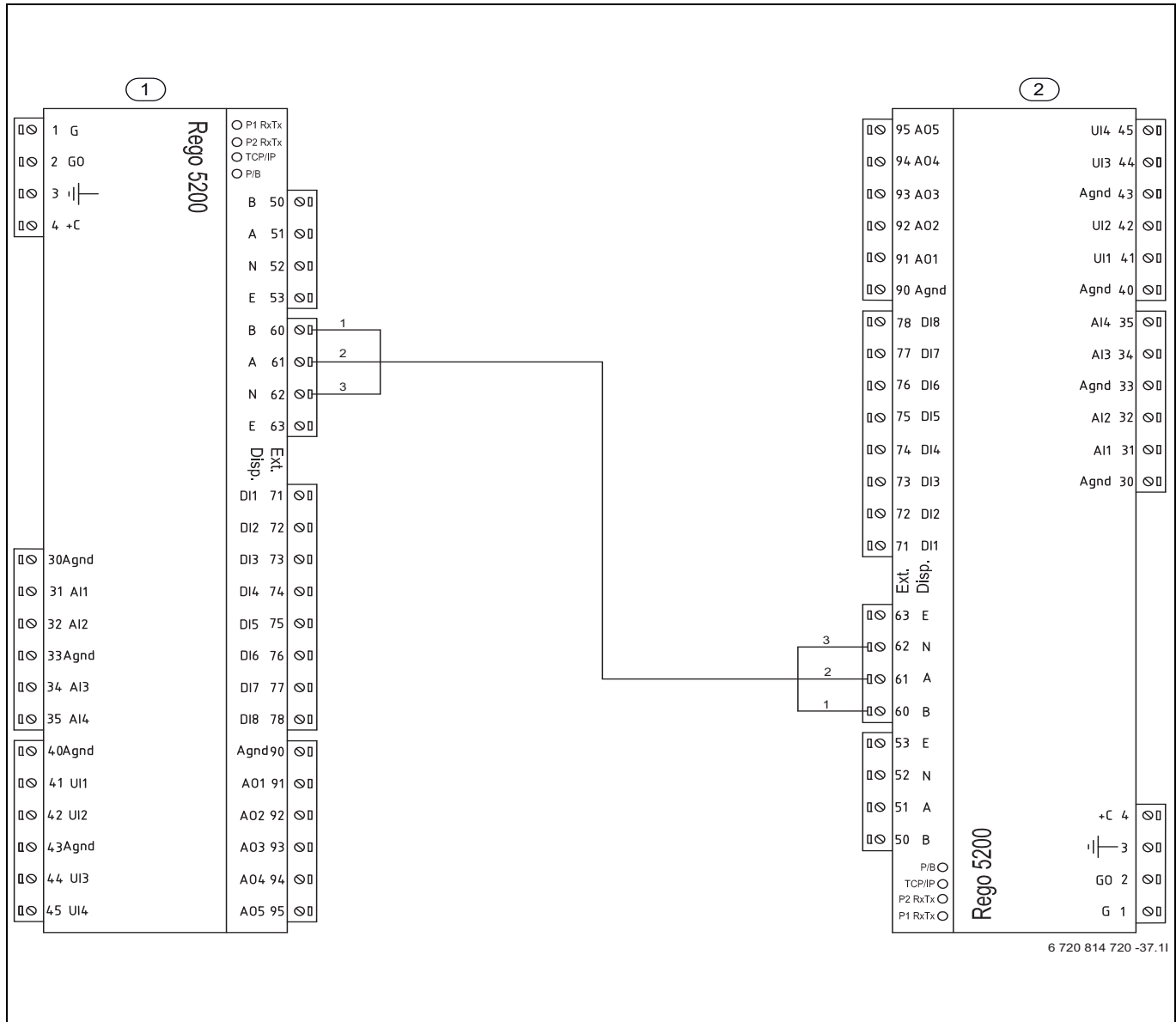
Kuva 21 Kaskadikytcentä 54–80 kW
