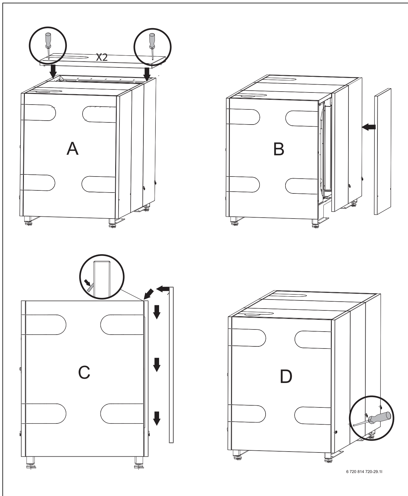
Kuva 8 Suojapeltien asentaminen/irrottaminen
