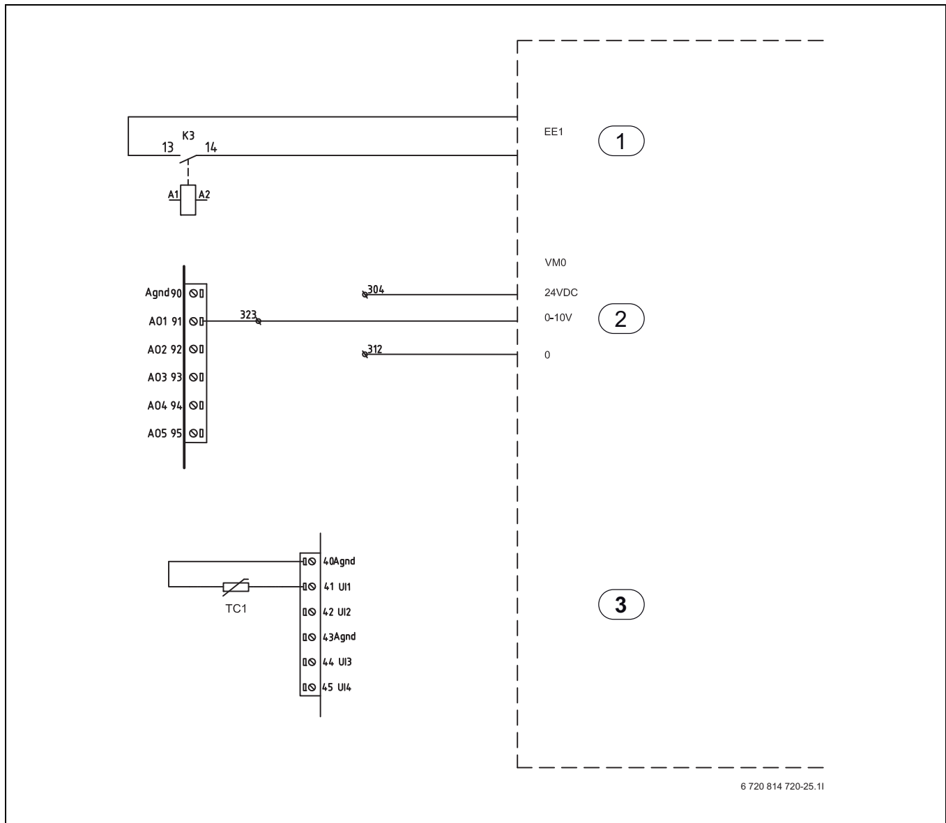
Kuva 44 Kytkenäkaavio, ulkoinen shuntattu lisälämpö
