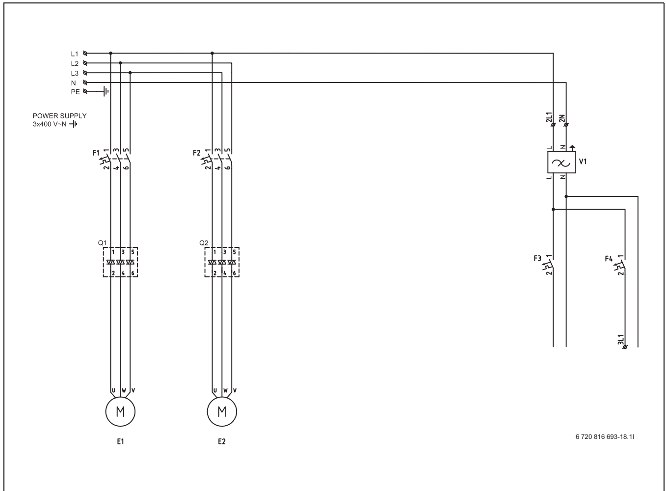
Kuva 38 Pääsyötön piirikaavio, lämpöpumppu 38–48 kW pehmökäynnistimellä (Q1/Q2)
