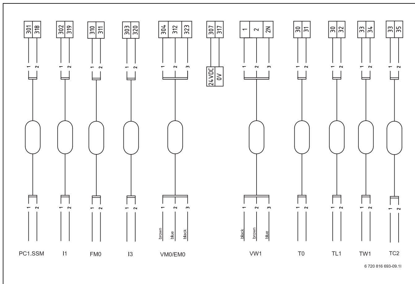
Kuva 36 Ulkoisten liitännöjen kytkentäkaavio, lämpöpumppu 38–48 kW
