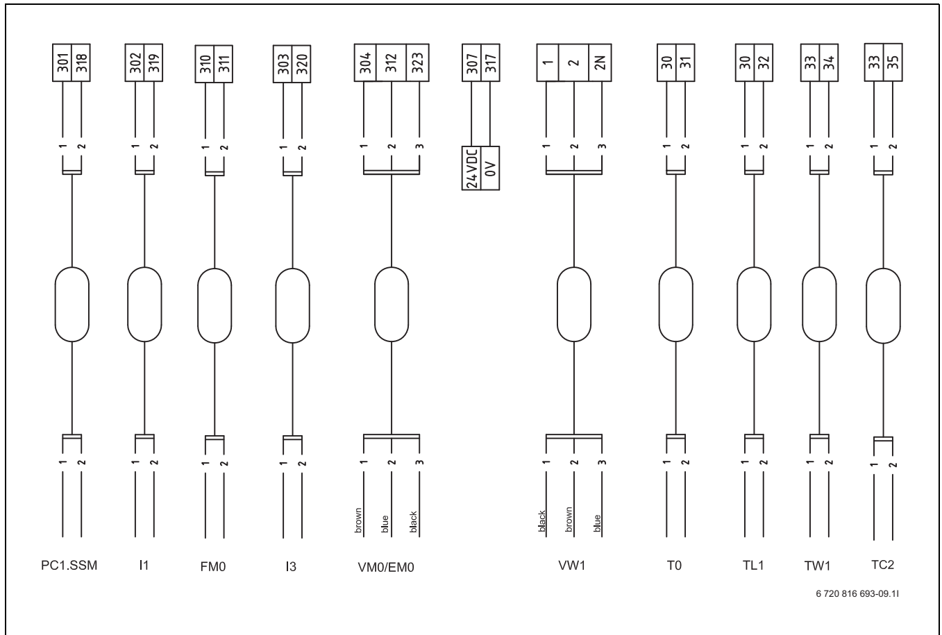
Kuva 36 Ulkoisten liitântöjen kytkentäkaavio, lämpöpumppu 38–48 kW
