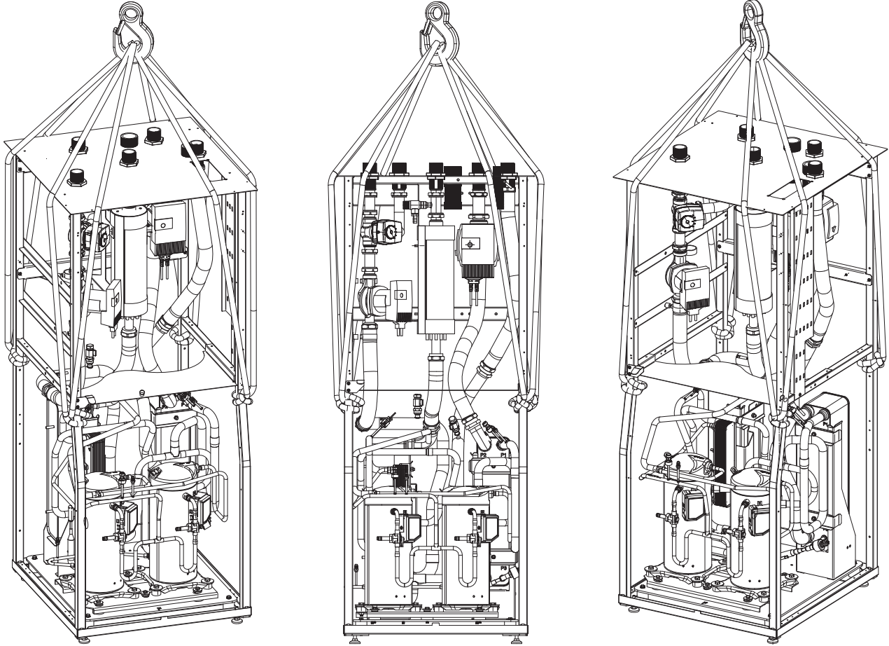
Kuva 3 Esimerkkejä 22–48 kW:n lämpöpumpun asennuksesta nostovöiden avulla.
