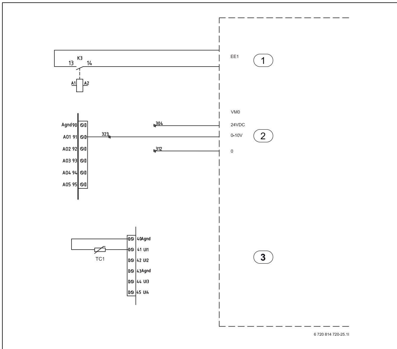
Kuva 44 KytKentäkaavio, ulkoinen shuntattu lisälämpö
